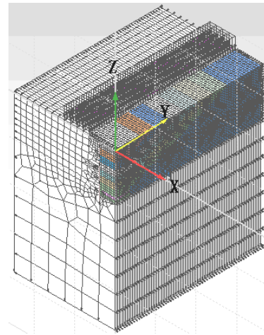
图 2 三维模型网格图
